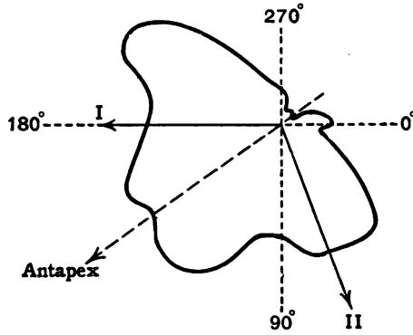
IX. Region XIV. ; centre R.A. 15^{\text{h}} 36^{\text{m}} , Dec. +17^{\circ} .
